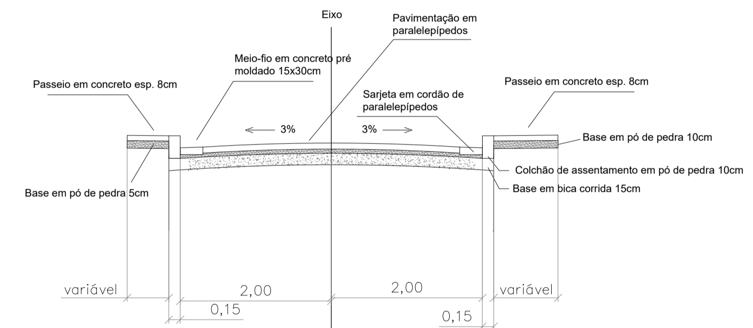
2 PERFIL TRANSVERSAL TIPO ESCALA: 1:50
